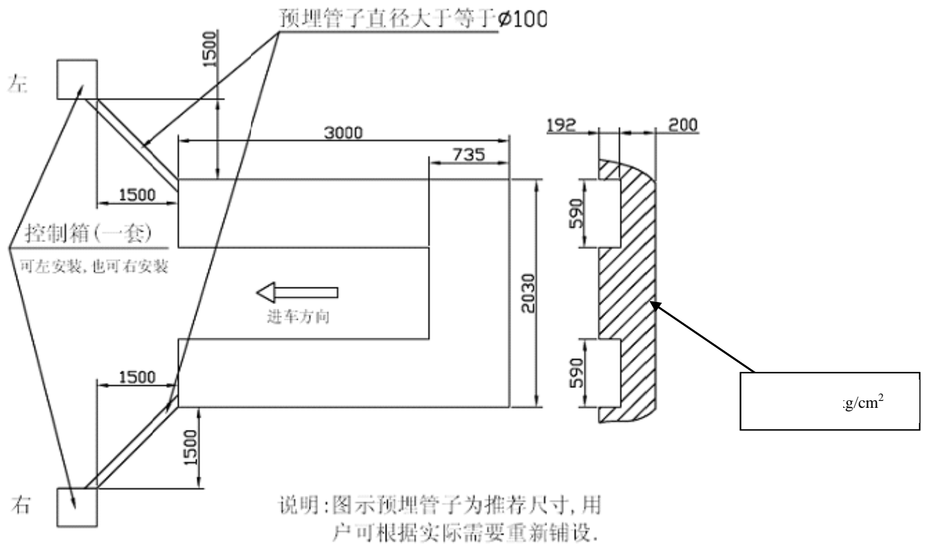
DS7000I-CN地基图
